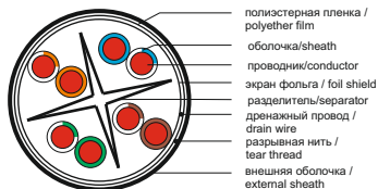
Рисунок 2 – конструкция кабеля типа F/UTP / Figure 2 – F/UTP type cable design
