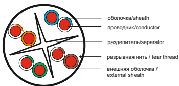
Рисунок 1 – конструкция кабеля типа U/UTP / Figure 1 – U/UTP type cable design
